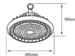
Potencia Ajustable
