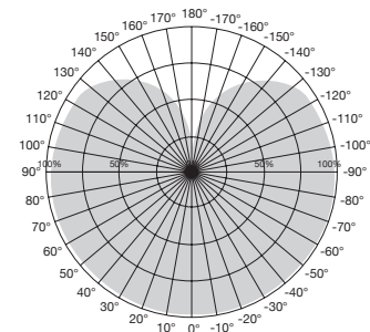
Beam Angle: 280°
