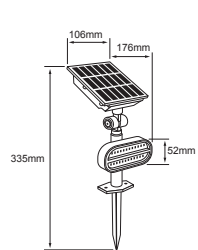
Doble aplicación: Estaca/ Sobreponer
