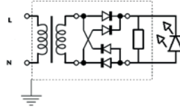
DIAGRAMA ELÉCTRICO: LED de 8.5 W
