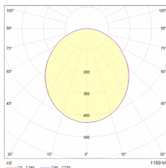
Unión T 100°
