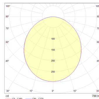
Unión L 100°
