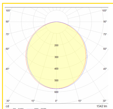
Unión X 100°
