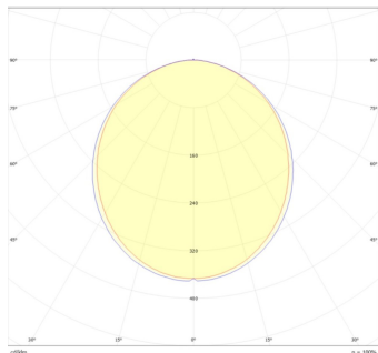
Magnettrack Pro Lineal 7W 110°
