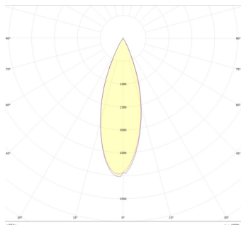
Magnettrack Pro Lineal Dirigible 15W 30°
