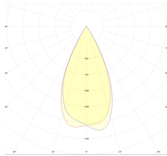
Magnettrack Pro Lineal Tipo proyector 12W 38°
