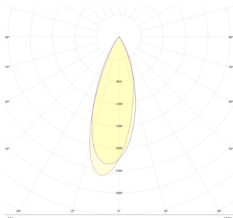
Magnettrack Pro Proyector 5W 30°
