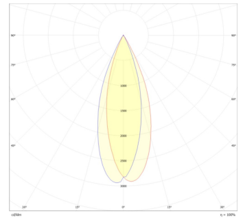
Magnettrack Pro Lineal Dirigible 10W 30°
