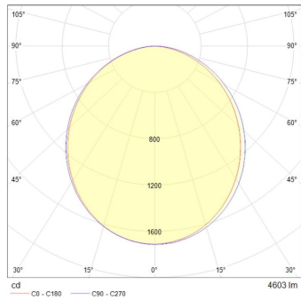
Unión 7 110°
