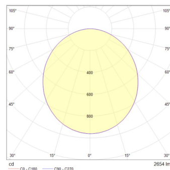
Unión X 110°
